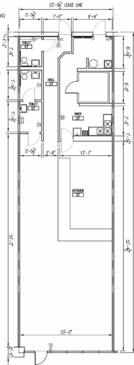
FLOOR PLAN SCALE: 1/8" = 1'-0"
