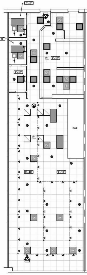
CEILING PLAN SCALE: 1/8" = 1'-0"
