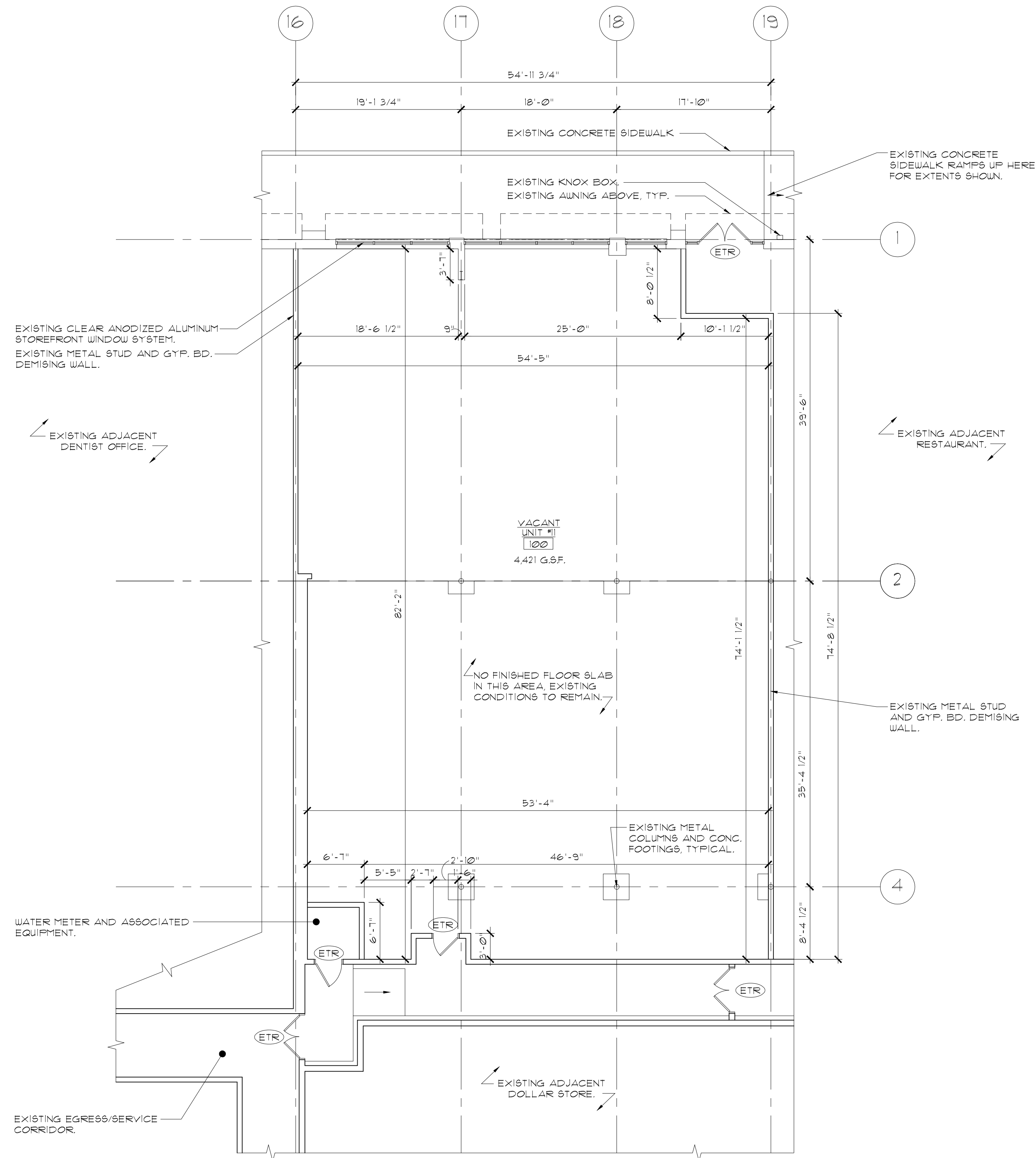
1 A-1 EXISTING FLOOR PLAN SCALE: 1/8" = 1'-0" N
